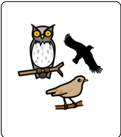
birds
