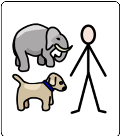
mammals
